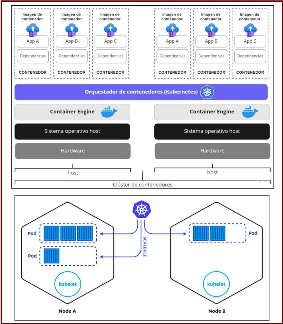
Entorno de contenedores + gestión mediante kubernetes
