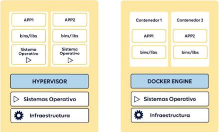
Máquina virtual vs. contenedor
