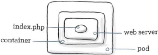
Contenedor + kubernetes
